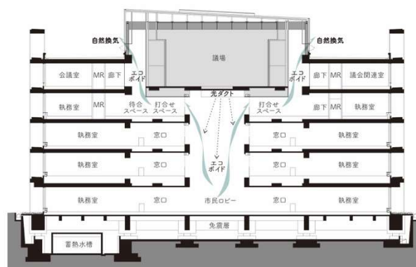
図-3 断面図
