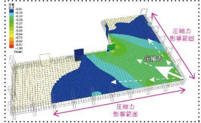
図-1-5 コーナー部に作用する付加圧縮力
