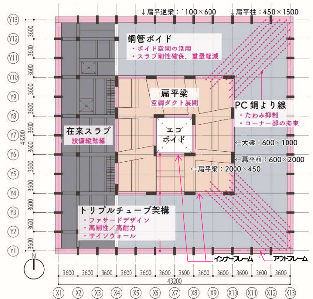
図-4 基準階伏図
