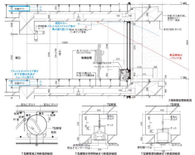
図-9 3階執務空間断面図
