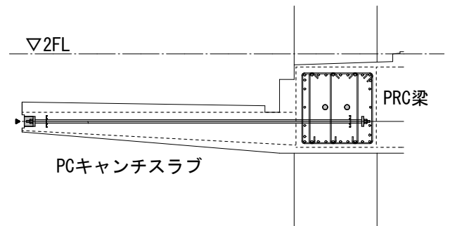
図-20 PRC梁とPCキャンチスラブの位置関係
