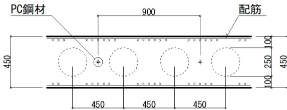
図-19 アンボンドボイドスラブ断面の一例
