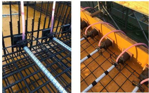
写真-13 PCキャンチスラブの配線状況 （左：固定定着具、右：緊張定着具）
