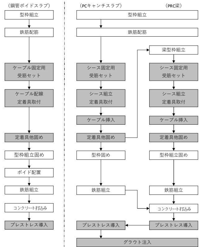
図-18 PC工事施工フロー
