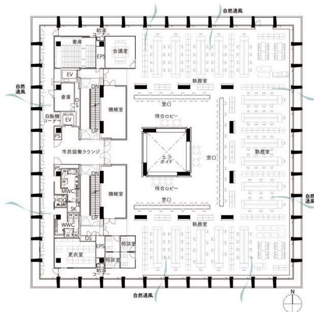
図-2 平面図
