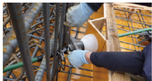
写真-8 三角形のヌスミを設ける
