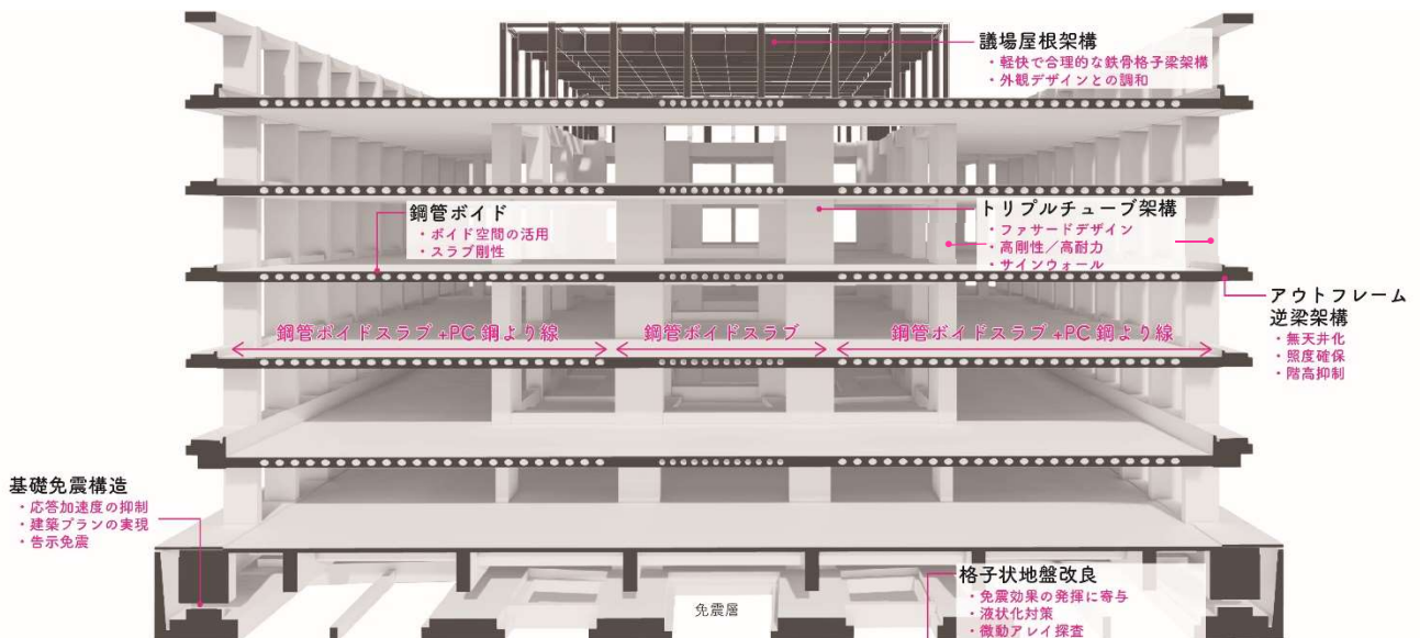
図-5 全体架構モデル
