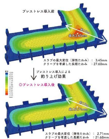
図-1-4 プレストレス導入による吊り上げ効果
