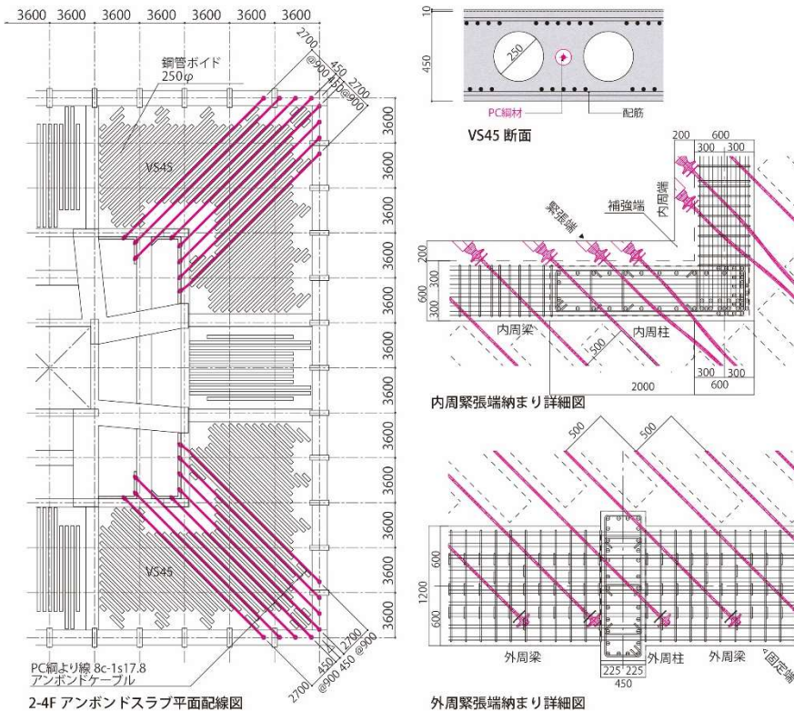
図-1-3 基準階コーナー部配線
