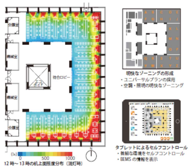
図-12 机上面照度分布
