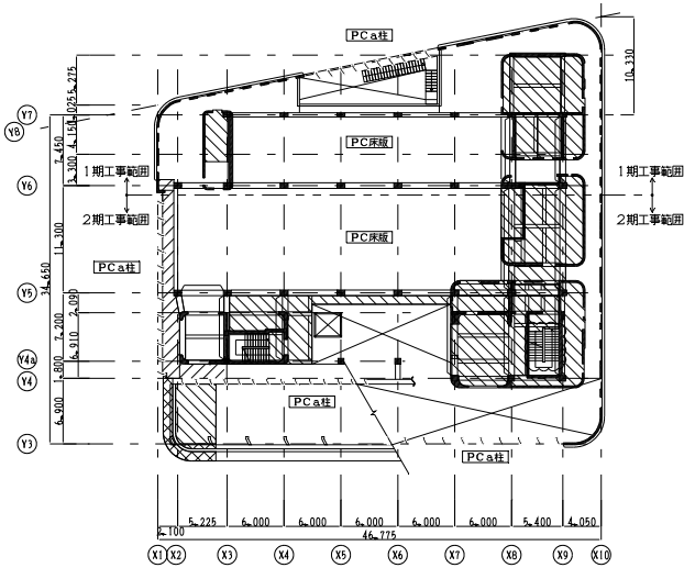
図-20 I期・II期工事範囲
