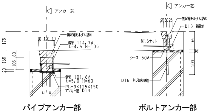
図-12 SU版 躯体接合詳細
