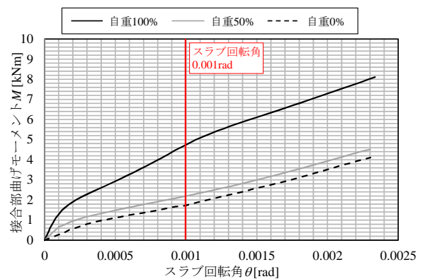
図-18 実験結果 ( M-\theta 関係)
