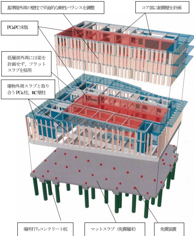
図-3 構造計画概念図
