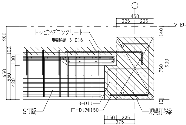
図-10 ST版 端部詳細図
