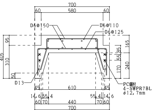
図-11 SU版 断面配筋形状
