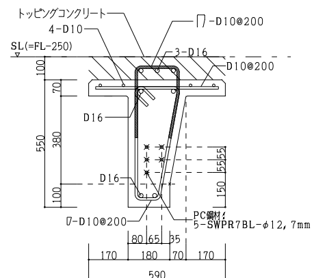
図-9 ST版 断面配筋形状 (一般階)
