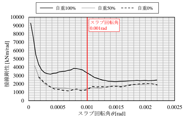
図-19 実験結果 (接線剛性)
