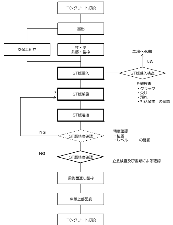
図-23 ST版施工フロー
