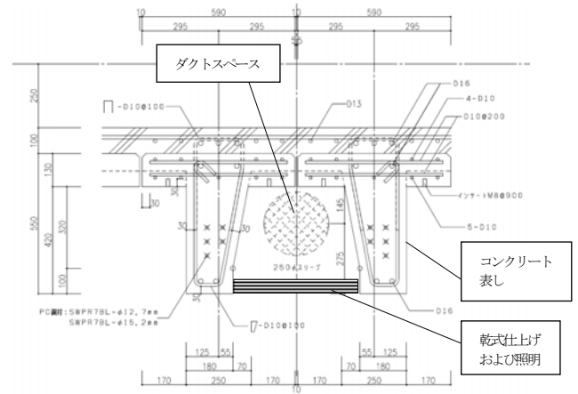
図-4 PCaPC 床版 (ST 版) の形状【一般部】
