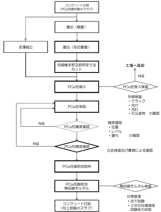
図-22 PCa柱施工フロー
