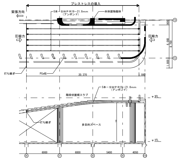
図-15 PC鋼材配線形状
