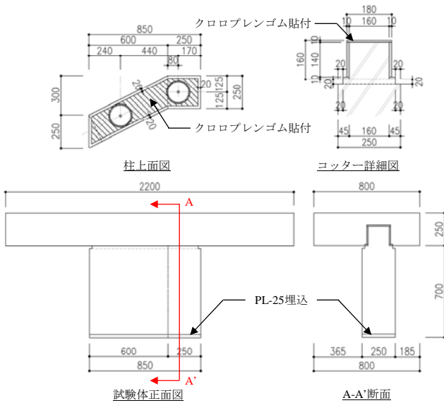
図-16 試験体詳細
