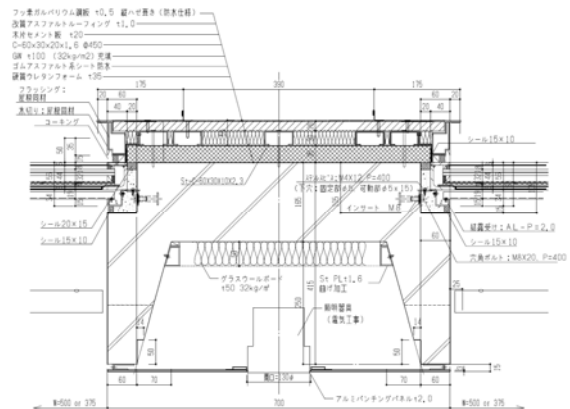
図-5 PCaPC 床版 (SU 版) の形状【議場】
