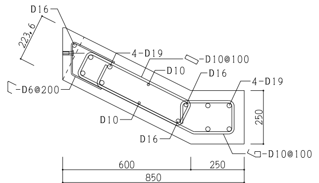
図-13 PCa柱 断面配筋形状
