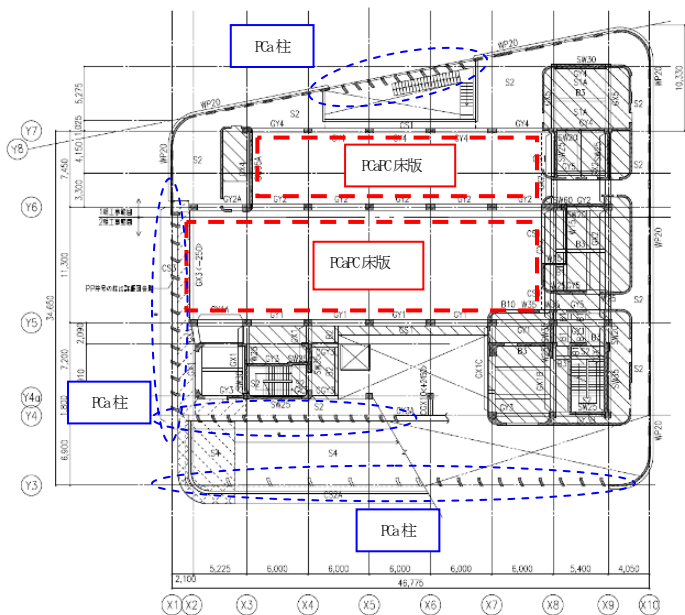
図-7 PCaPC 床版、PCa 柱の配置
