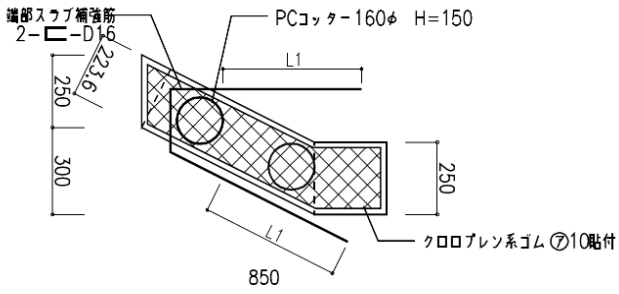
図-14 PCa柱 柱頭ピンディテール詳細図
