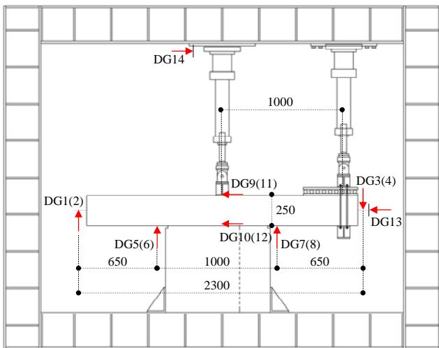
図-17 荷装置
