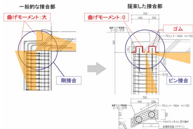
図-6 PCa 柱の柱頭ピンディテール概念図
