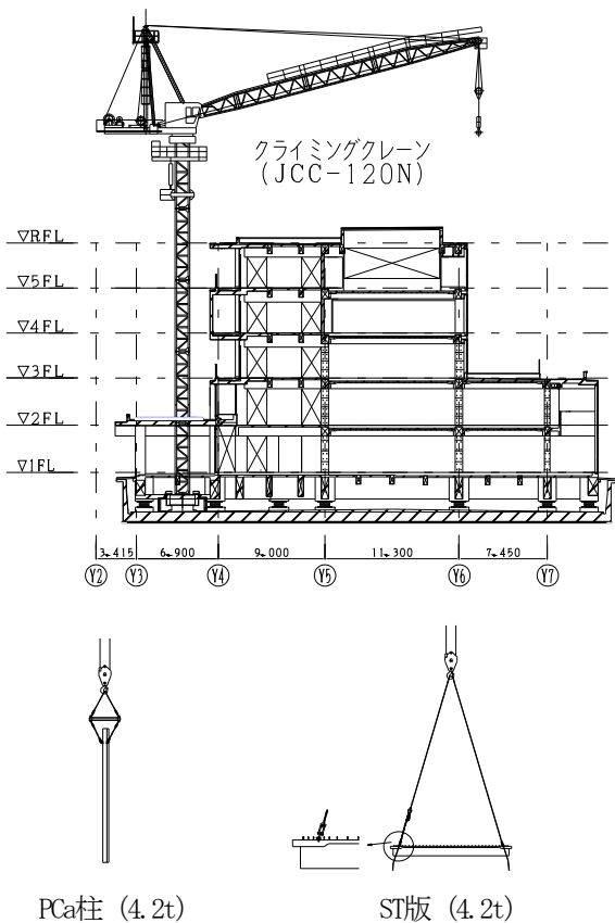
図-21 II期工事揚重計画図
