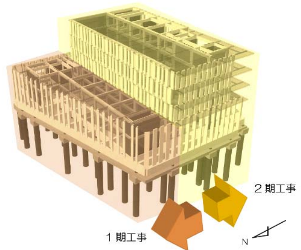
図-8 1,2期の工事範囲図
